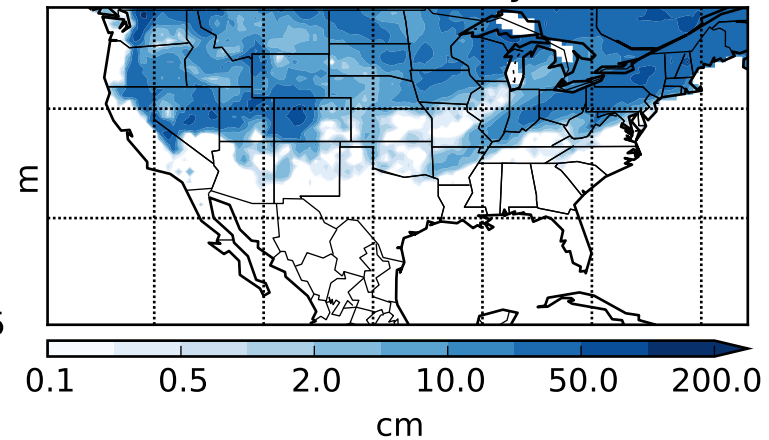
E2O Snow Analysis
